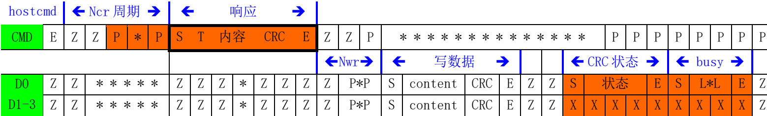
图 4-31：单块写命令时序
