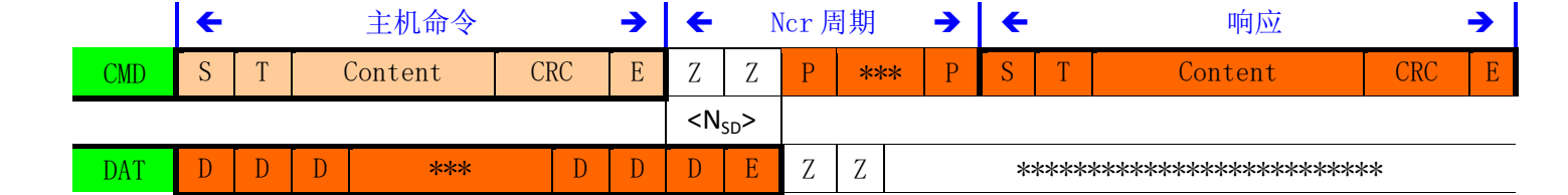
图 4-30：停止命令时序 (CMD12，数据传输模式)
