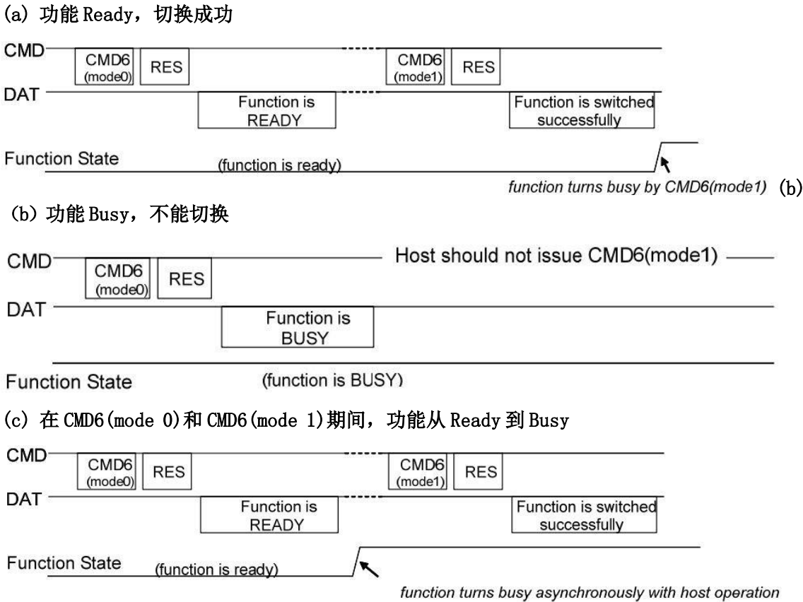
图 4-18 切换功能流程实例
