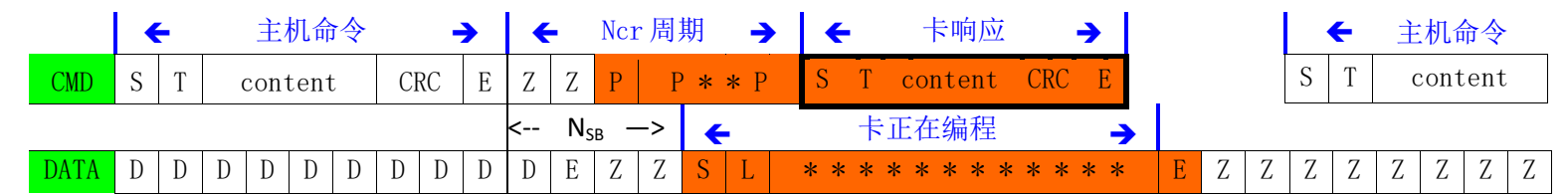
图 4-33：主机数据传输期间停止传输
