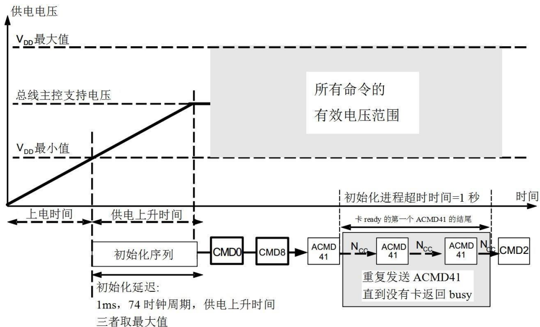
图 6-4 上电流程
