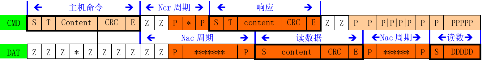
图 4-29：多块读命令时序
