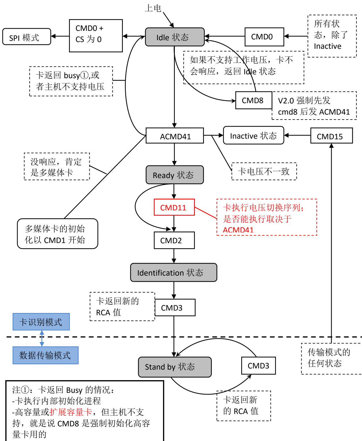
图 4-1 SD 卡识别模式状态图
